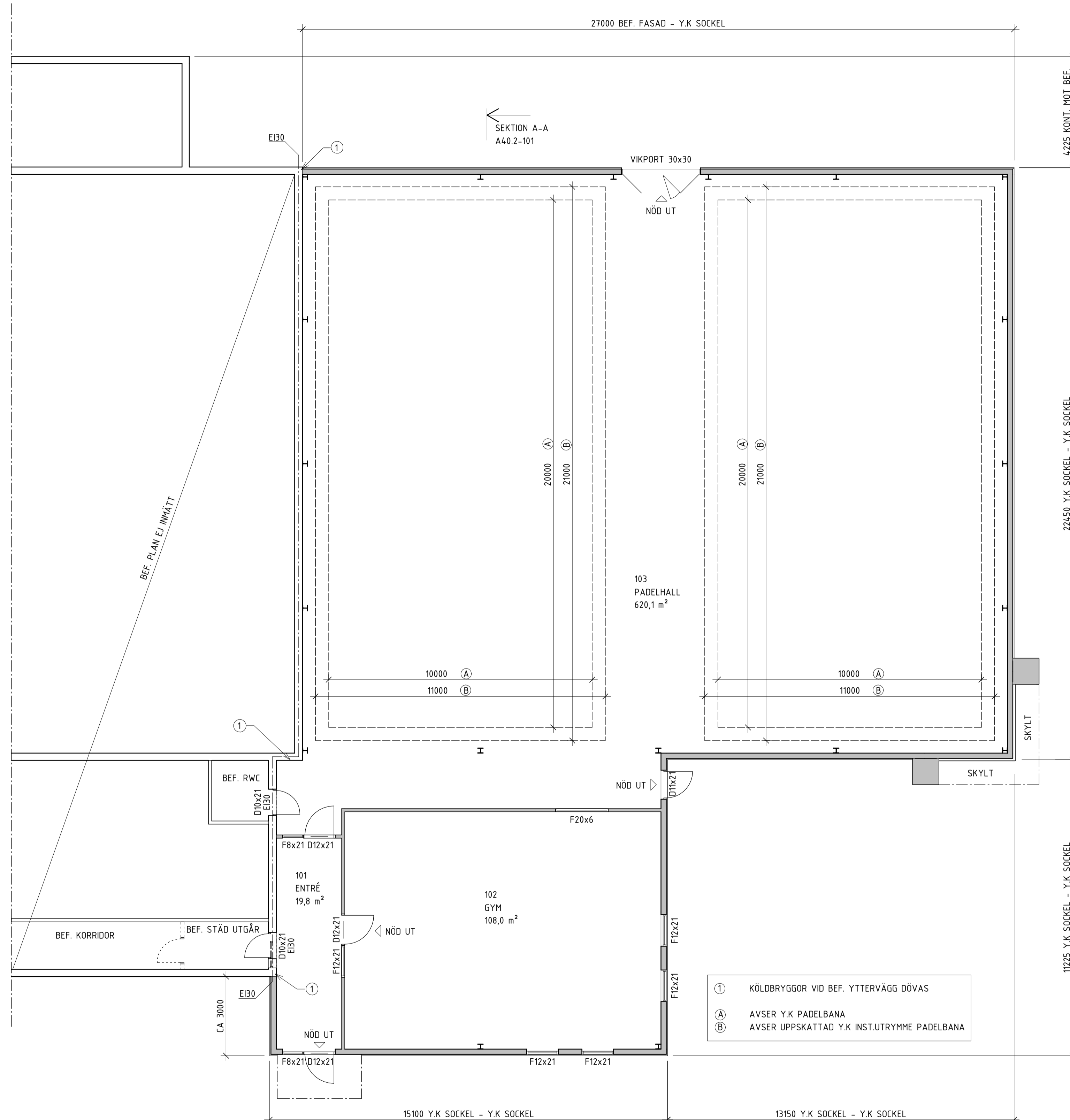
-PLAN -1:100- (A1)
